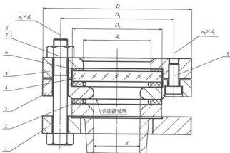
图2 B型搪玻璃带视镜手孔
