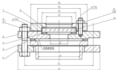
图 1 A 型搪玻璃带视镜手孔
